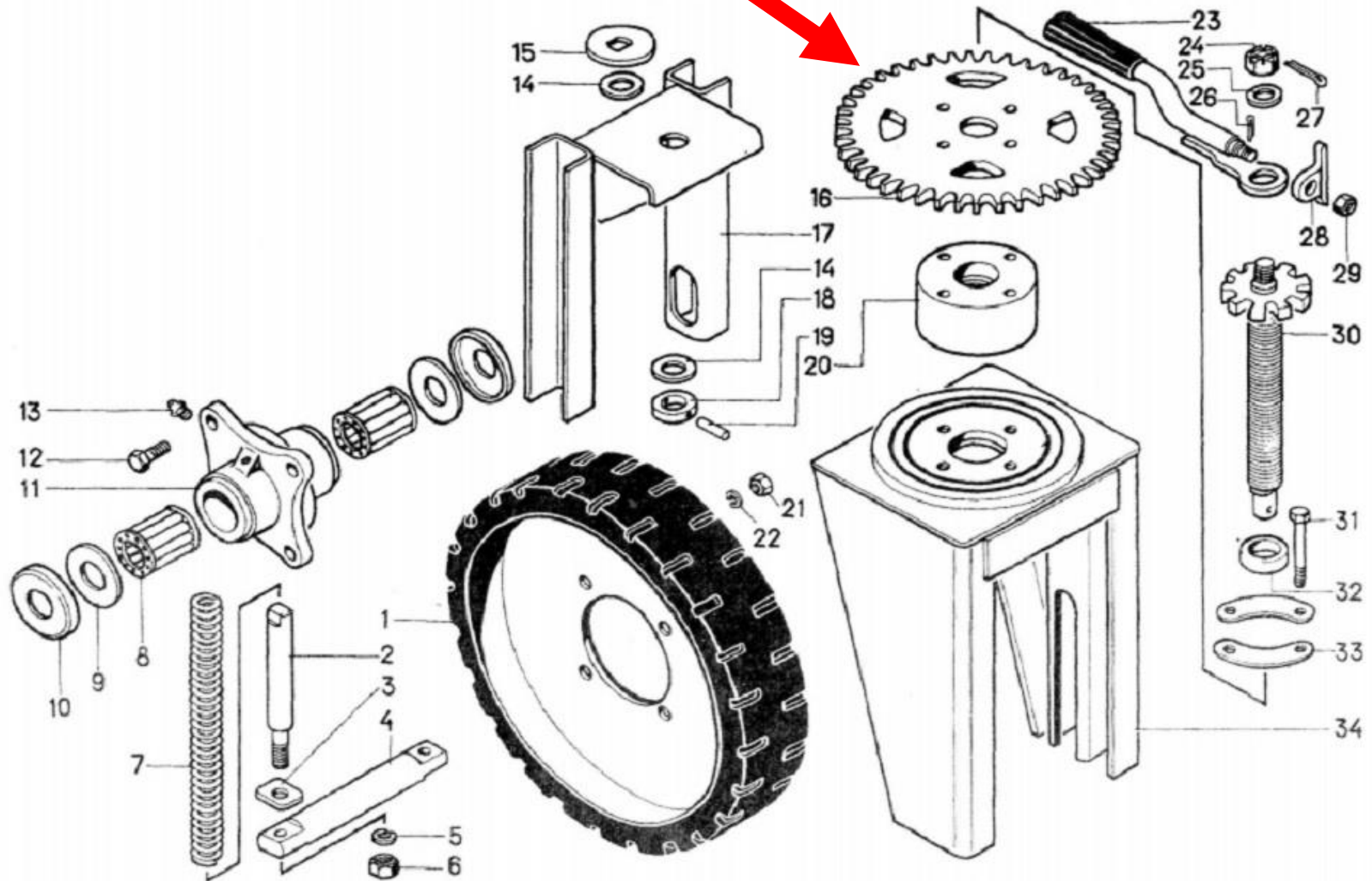
Рис. 4. Ход передний ЗП 01.020
